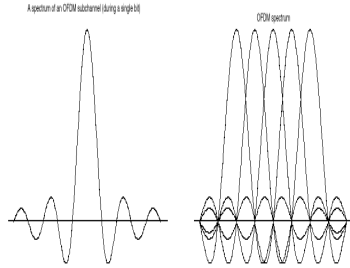
Fig. 1 OFDM SPECTRUM
